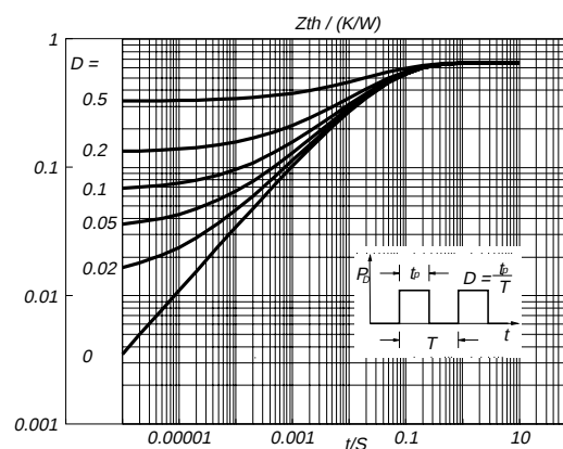
Fig.4. Transient thermal impedance. Z_{th j-mb} = f(t) ; parameter D = t_p / T
